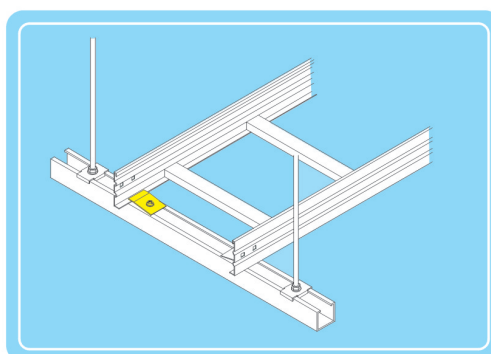
內側固定片 INSIDE HOLD DOWN CLIP
